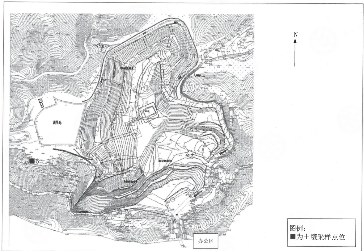
图 5-1 土壤布点图
