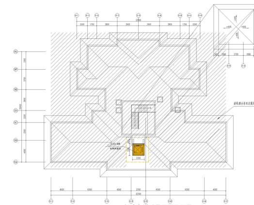
加建电梯后屋面层平面图
