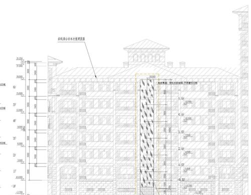
加建电梯后 ④-⑤轴立面图
