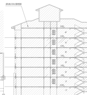
加建电梯后A-A剖面图
