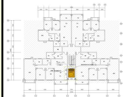
加建电梯后二层平面图
