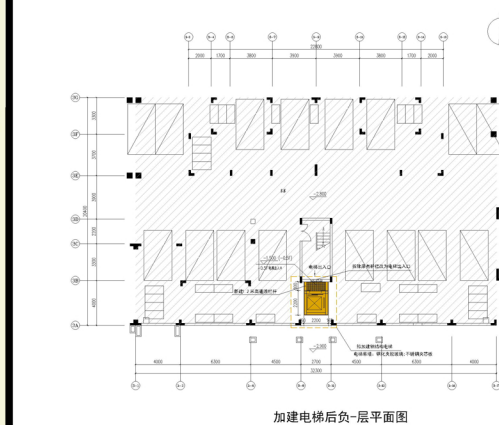
加建电梯后负一层平面图
