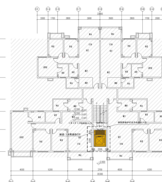
加建电梯后三至六层平面图
