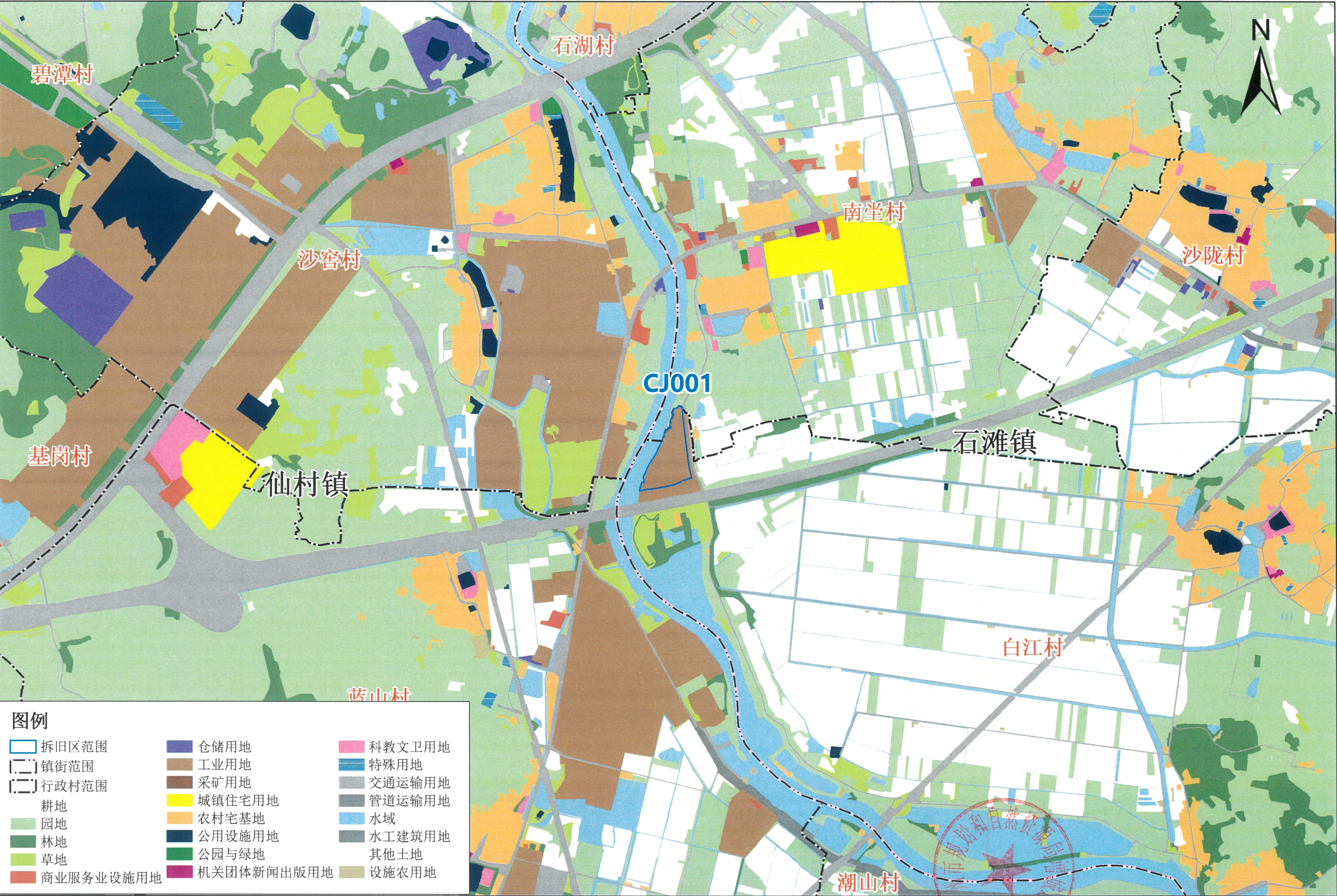
增城区城乡建设用地增减挂钩石滩镇南埗村、郑田村项目区（全域土地综合整治）拆旧区土地利用现状图（2023年）
