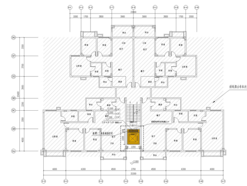
三-六层平面图
