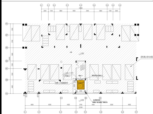
首层平面图
