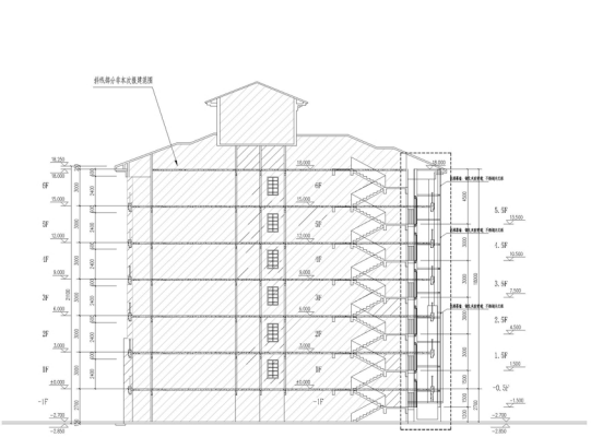
A-A剖面图
