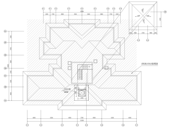
天面层平面图
