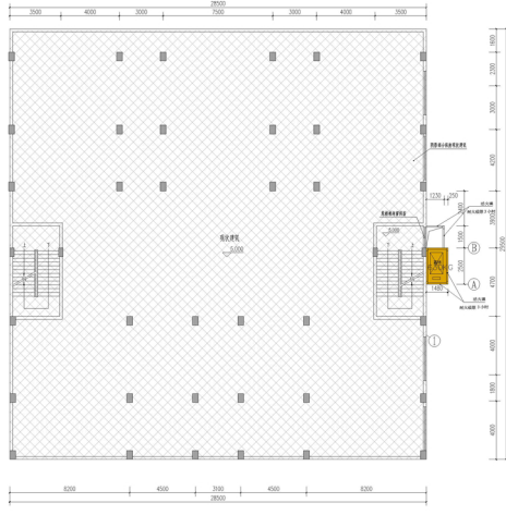
二层平面图
