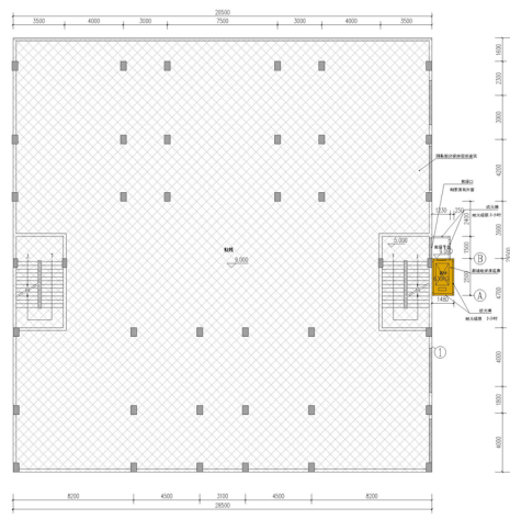
三层平面图
