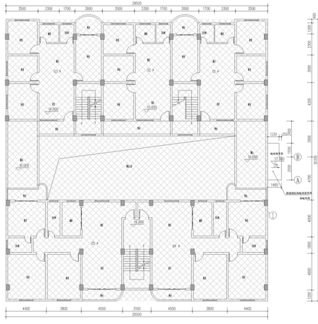
五层(电梯井天面层)平面图
