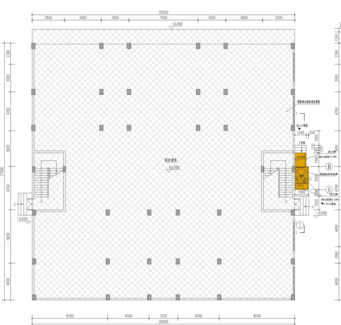
首层平面图
