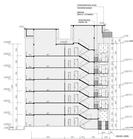
1-1剖面图
