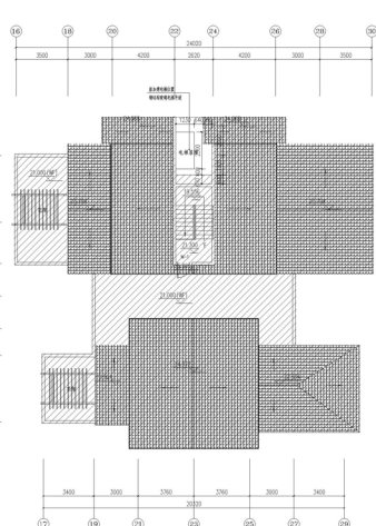
天面层平面图
