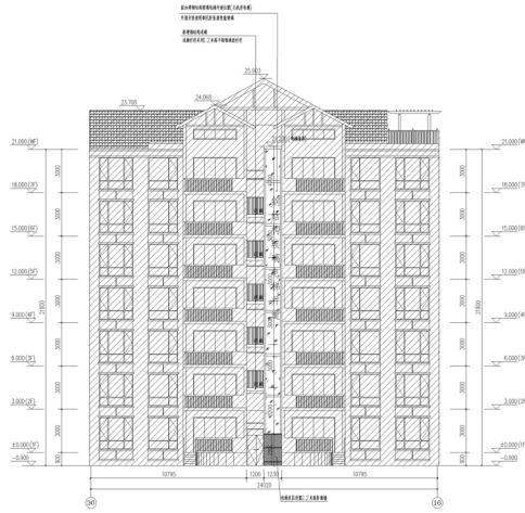
立面图
