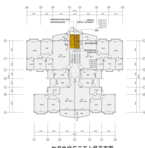
加装电梯后三至七层平面图
