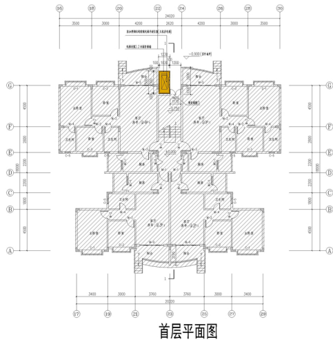
首层平面图
